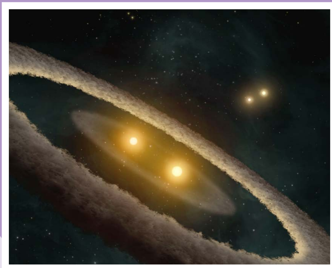
Двойные звёзды
