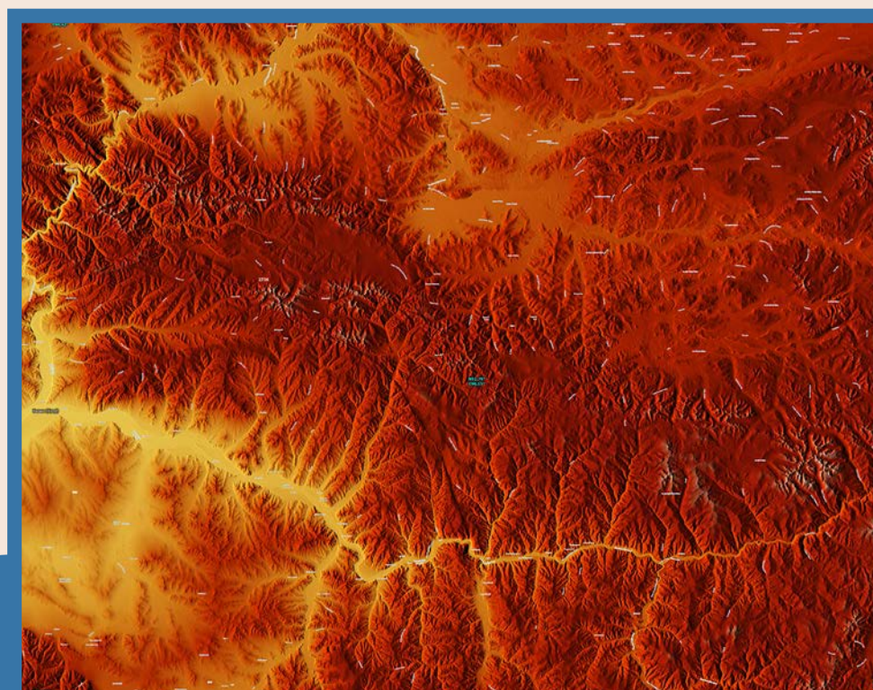
Хребет Обручева. Республика Тува. Спутниковый фотоснимок
