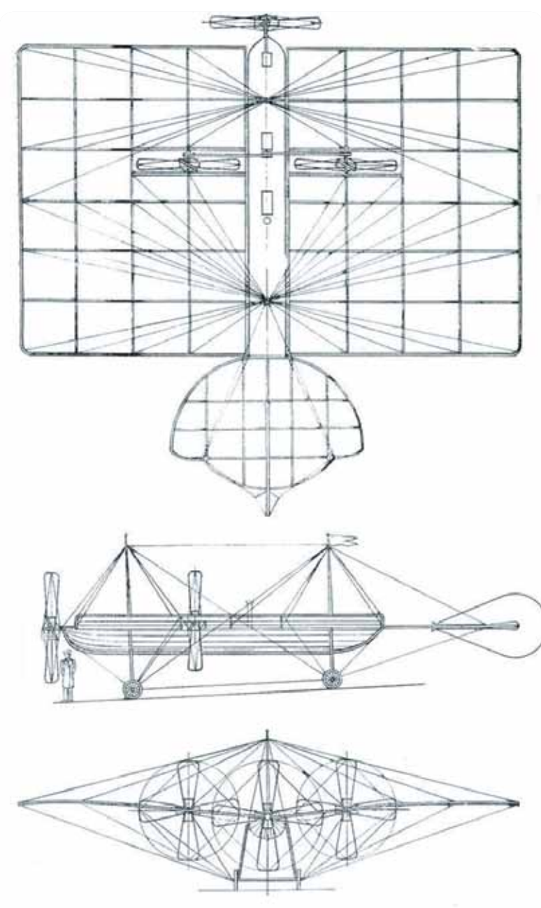
Чертеж моноплана Можайского
