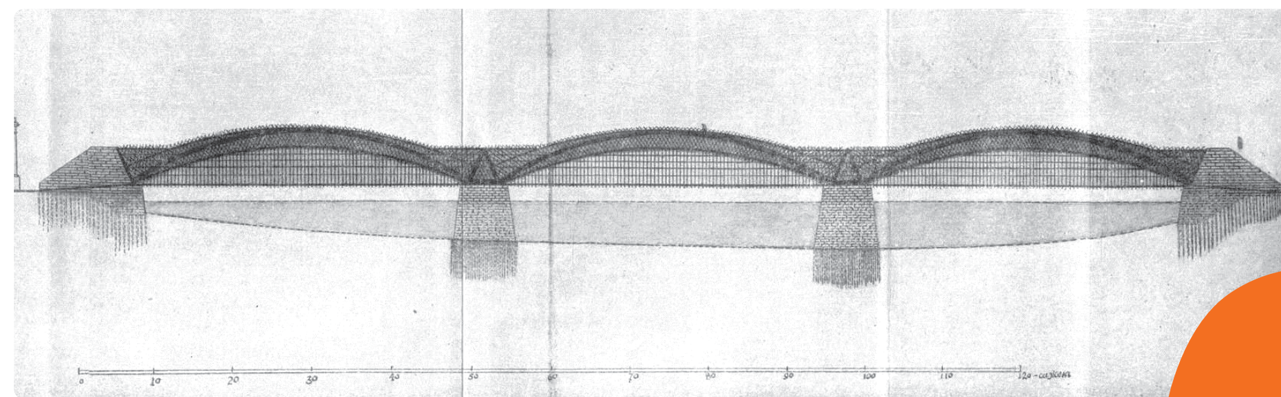
Проект моста через Неву
