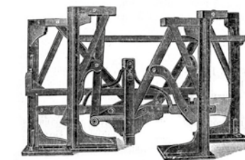
Модель стопходящей машины П. Л. Чебышёва
