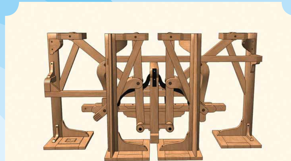
Модель «стопходящей машины»
